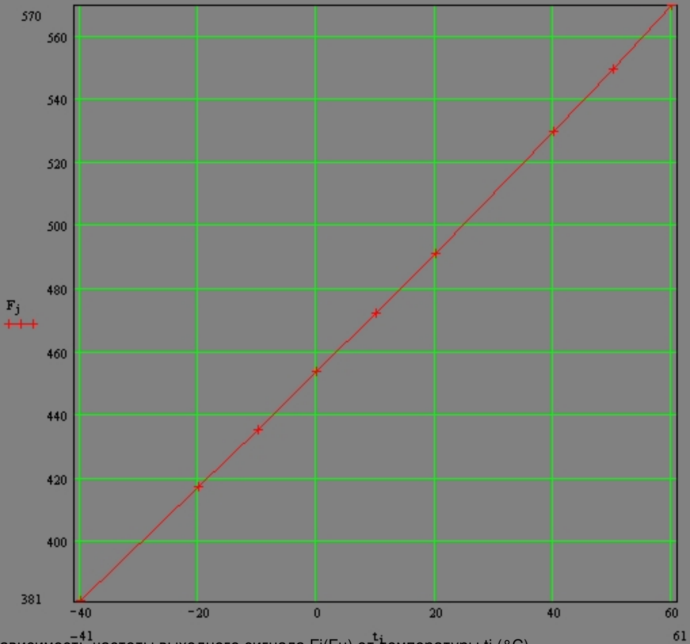
Зависимость частоты выходного сигнала F_j (Гц) от температуры t_j (°C)
