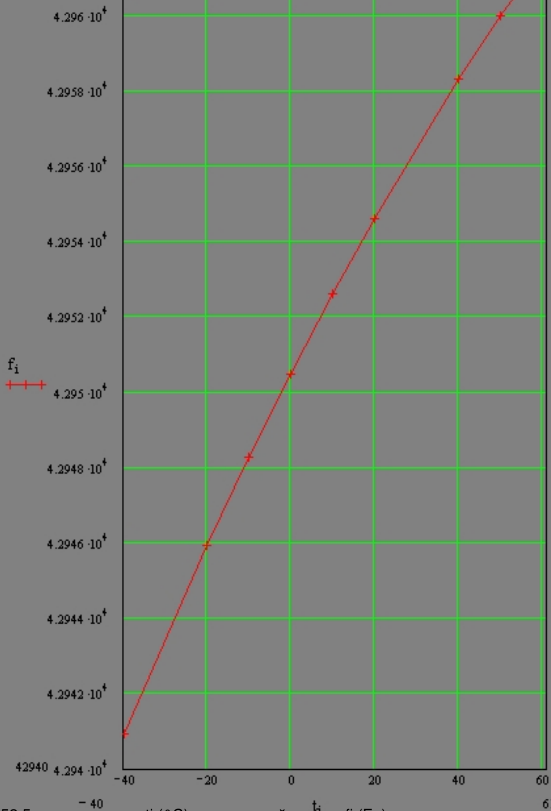
Влияние температуры t_i (°C) на выходной сигнал f_i (Гц) при постоянном давлении
